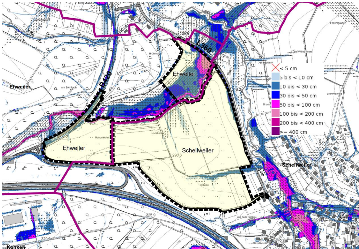
Abbildung 5 Sturzflutgefahrenkarte des Landesamtes für Umwelt Rheinland-Pfalz (Wassertiefen SR17, 1h), November 2025
